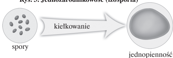
Rys. 3. Jednozarodnikowość (izosporia)
