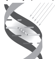
3. Zablockowanie replikacji
